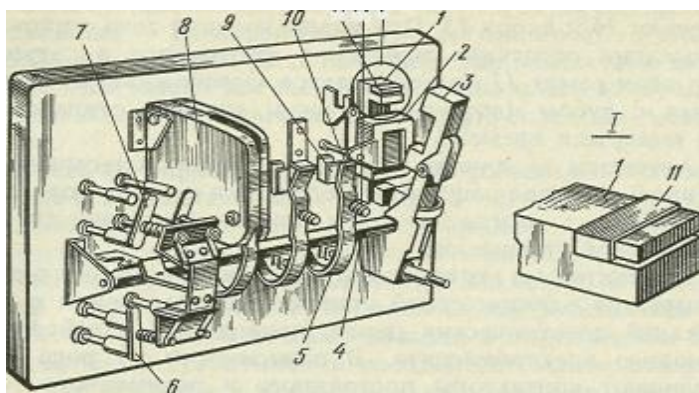
Рис. 6 Трехполюсный контактор переменного тока: / — ярмо, 2 — катушка, 3 — якорь, 4 — вал, 5 — соединение подвижного контакта, 6, 7 — блок-контакты, 8 — дугогасительная камера, 9, 10 — контакты, 11 — коротко-замкнутый виток, 12 — пружина
