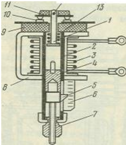
Рис. 8 Максимальное реле: 1 - стержень, 2 - трубка, 3 - скоба, 9 - изолирующая колодка, 10 - контакты, 11 - коромысло, 12 - ось, 13 – пружина
