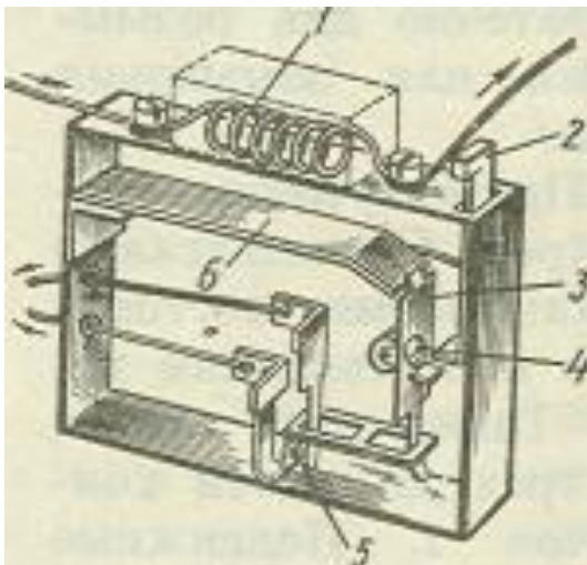
Рис. 9 Тепловое реле: 3 -рычаг, 4 - пружина, 5 - контакты, 6 – биметаллическая пластина
