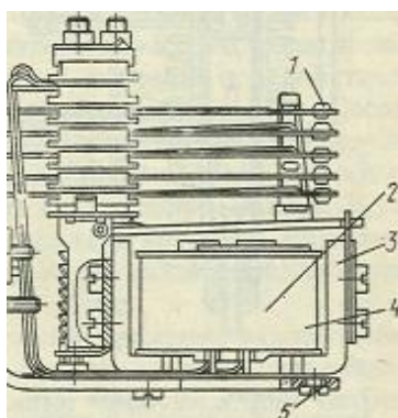
Рис. 7 Промежуточное реле:
