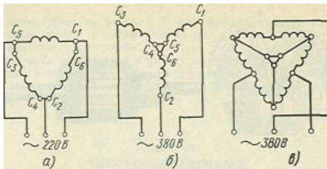
Рис. 2. Схемы соединения обмоток статора асинхронных электродвигателей:
