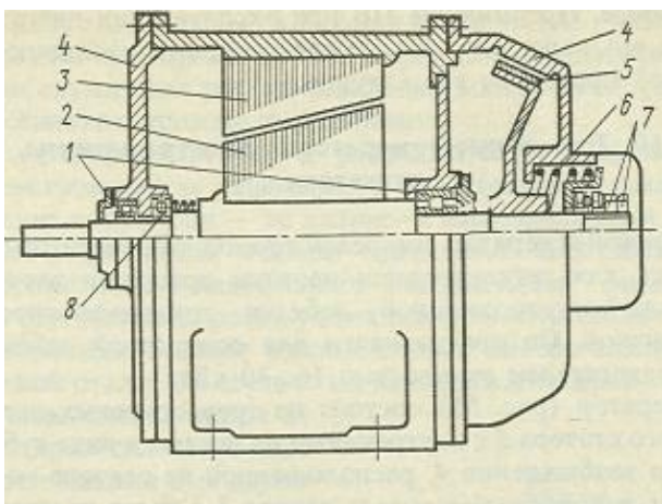
Рис. 3 Самотормозящий электродвигатель
